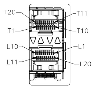
DETAIL A 1:1
